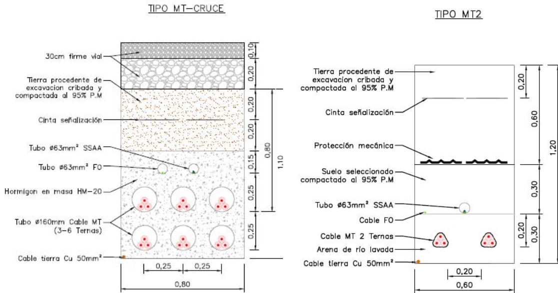
Ilustración 3: Zanjas MT
